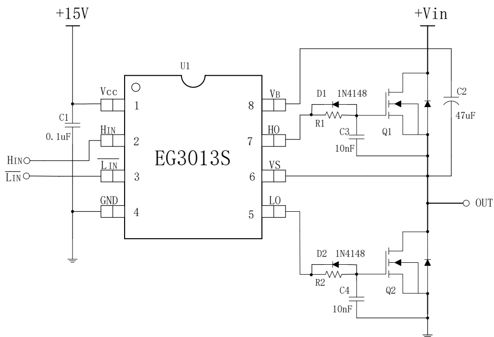
图 6-1. EG3013S 典型应用电路图——中、小功率半桥驱动应用
