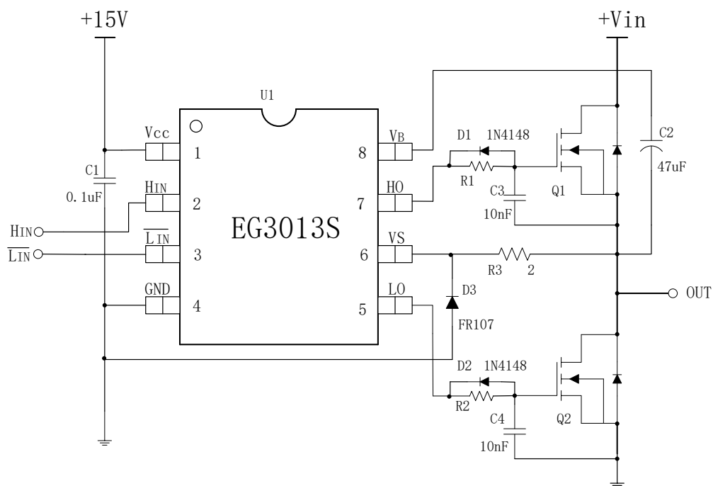
图 6-2. EG3013S 典型应用电路图——大功率电机场合应用
