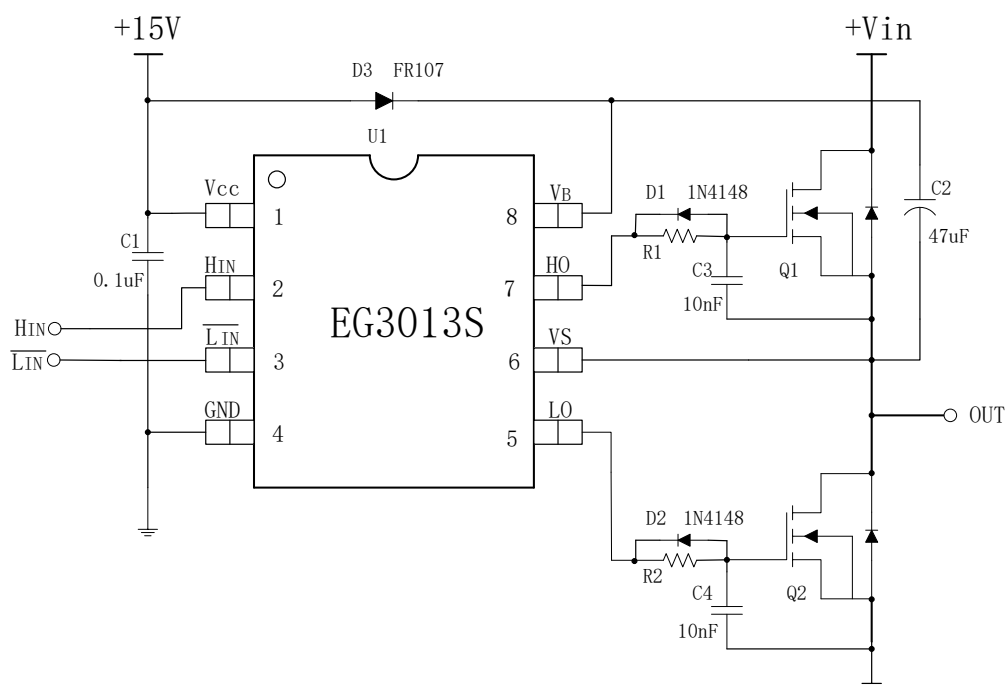
图 6-3. EG3013S 典型应用电路图——外接自举二极管应用
