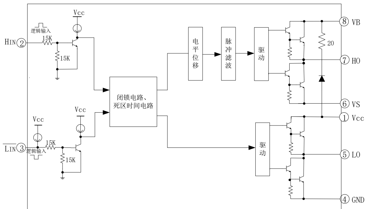
图 5-1. EG3013S 结构框图
