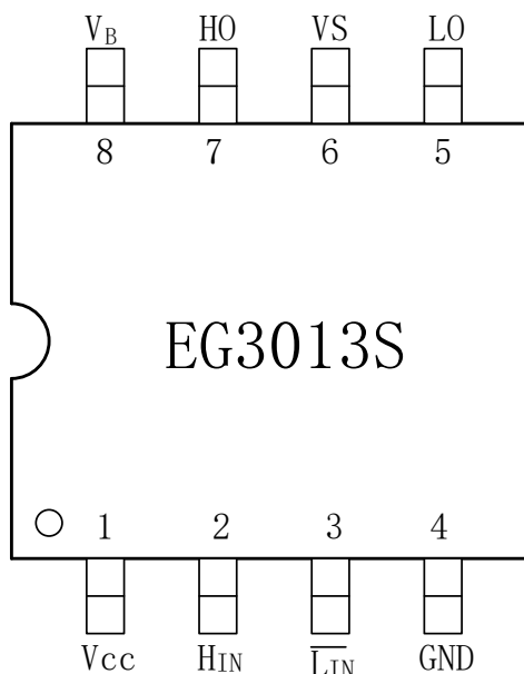
图 4-1. EG3013S 管脚定义
