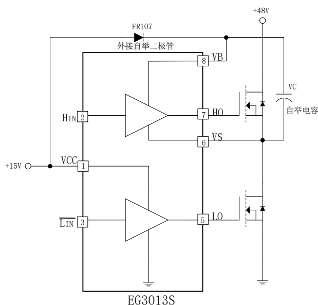
图 8-3. EG3013S 自举电路结构
