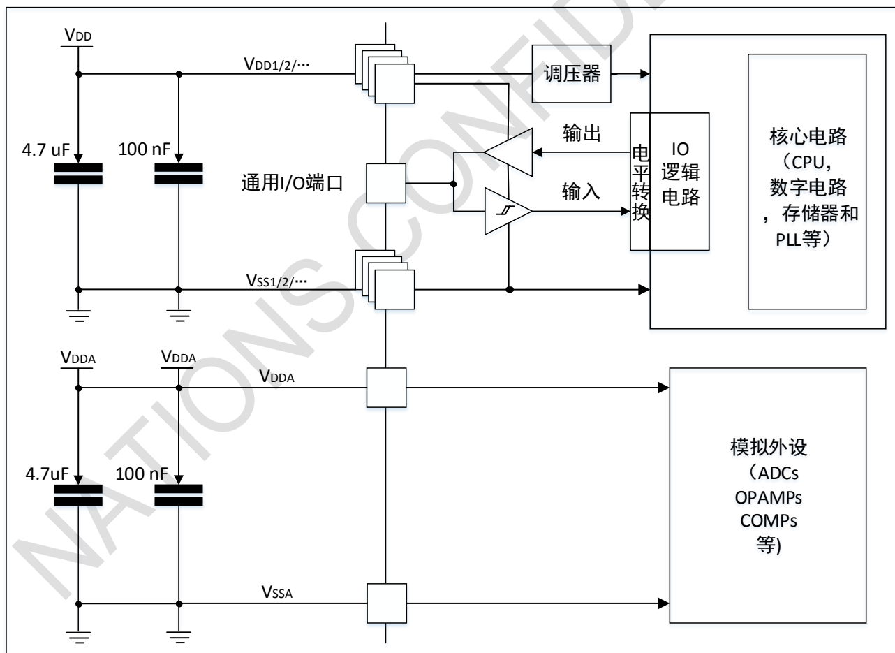
图 4-3 供电方案
