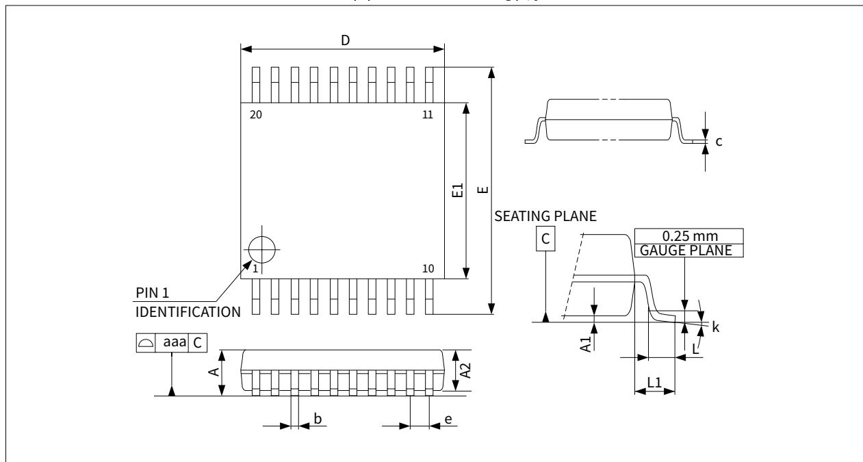
图 8-5 TSSOP20 引线
