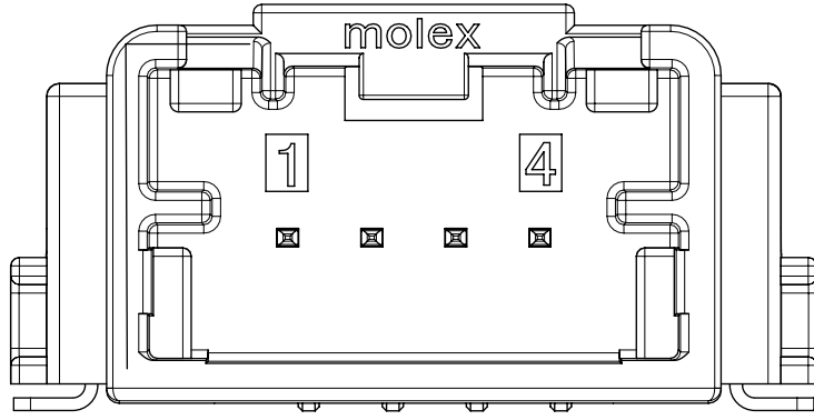
4 CKT SMT HEADER POLARIZATION OPTION A
