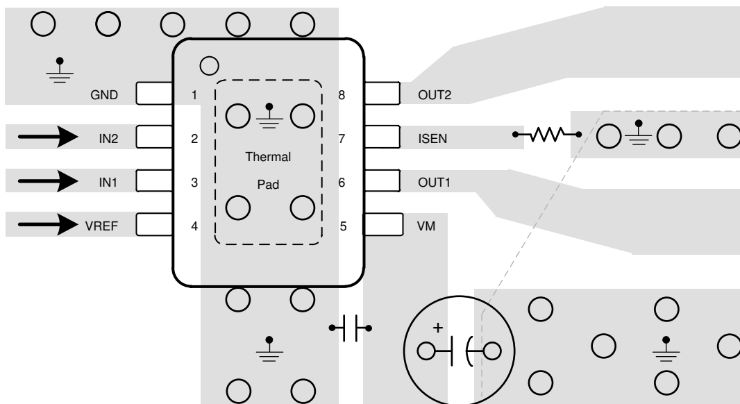
图 11-2. Layout Recommendation
