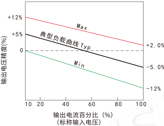
误差包络曲线图 3.3Vdc输出
