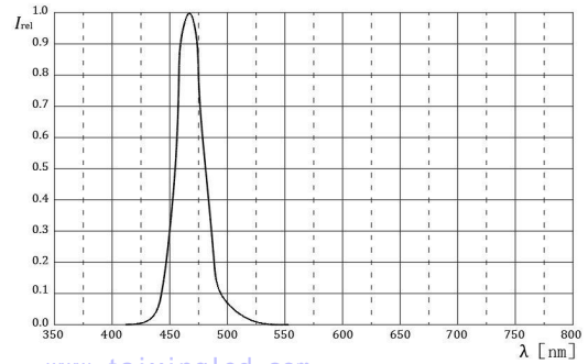
Relative Spectral Emission 相对光谱发射 IF=20mA, Ta=25°C
