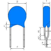
前后翘脚型引线
