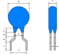
青蛙脚型引线
