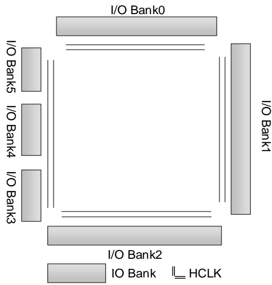
图 2-22 GW1N-4 HCLK 示意图
