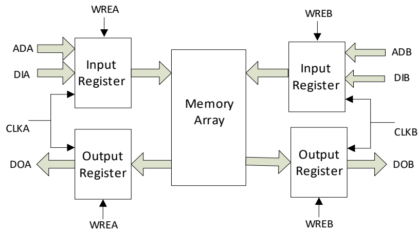
图 2-17 独立时钟模式
