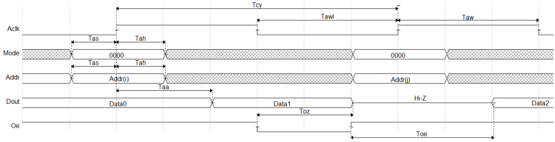
图 3-1 读操作模式
