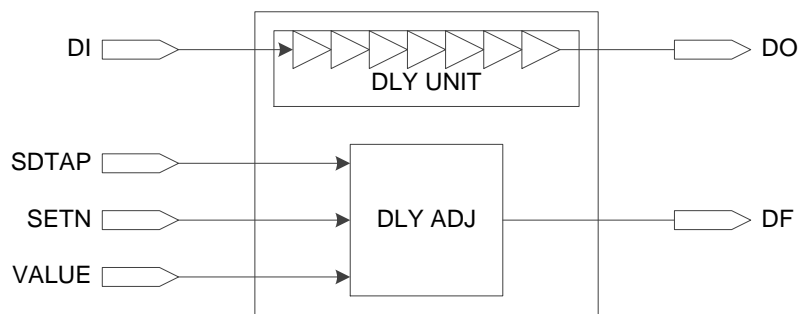
图 2-6 IODELAY 示意图
