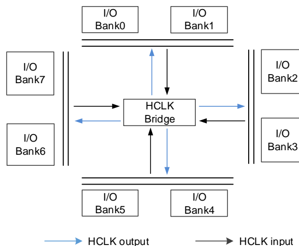
图 2-14 GW2A 系列 FPGA 产品的 HCLK 示意图
