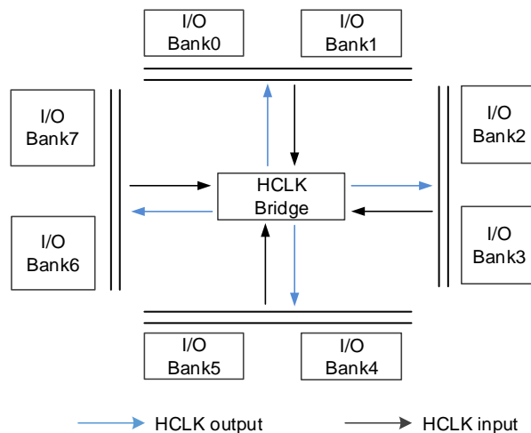
图 2-14 GW2AR 系列 FPGA 产品的 HCLK 示意图
