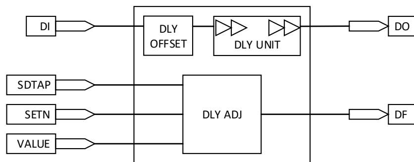
图 2-11 IODELAY 示意图
