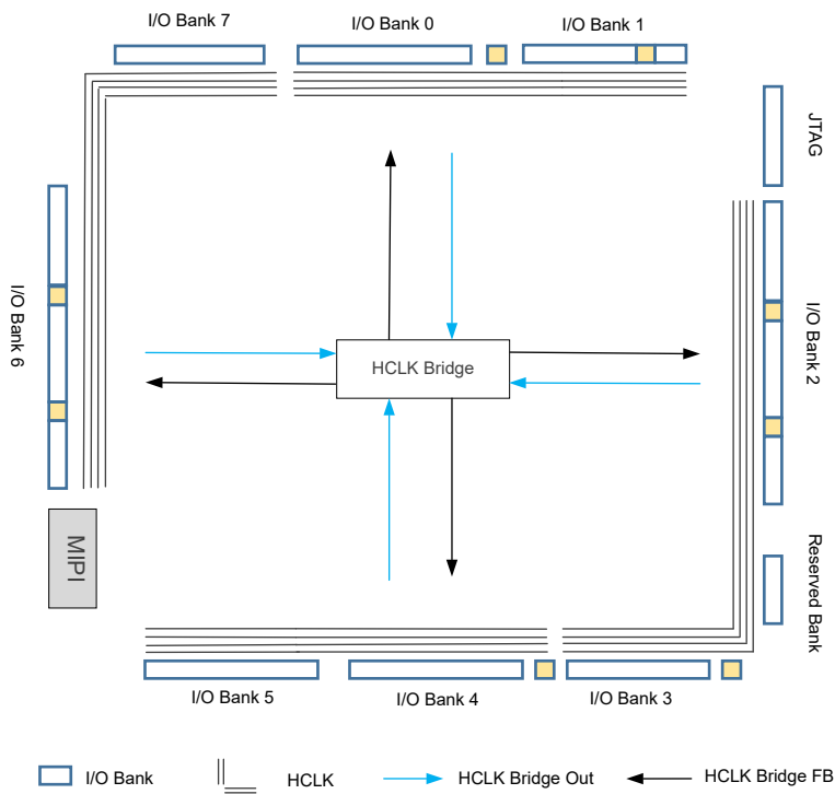
图 2-18 HCLK 示意图(GW5A-25)
