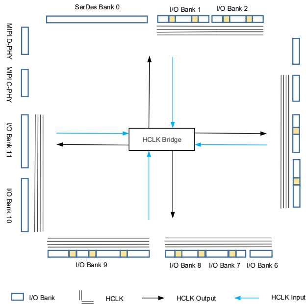
图 2-18 HCLK 示意图(GW5A-25)
