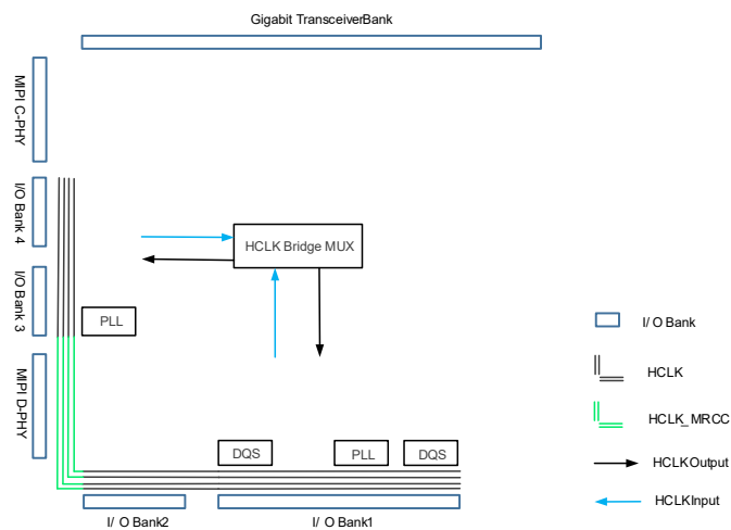
图 2-23 HCLK 示意图(GW5AT-15)
