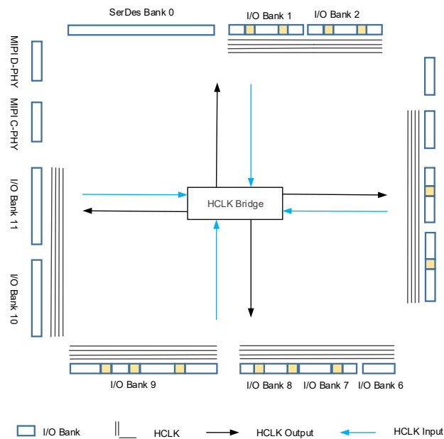
图 2-23 HCLK 示意图(GW5AT-15)
