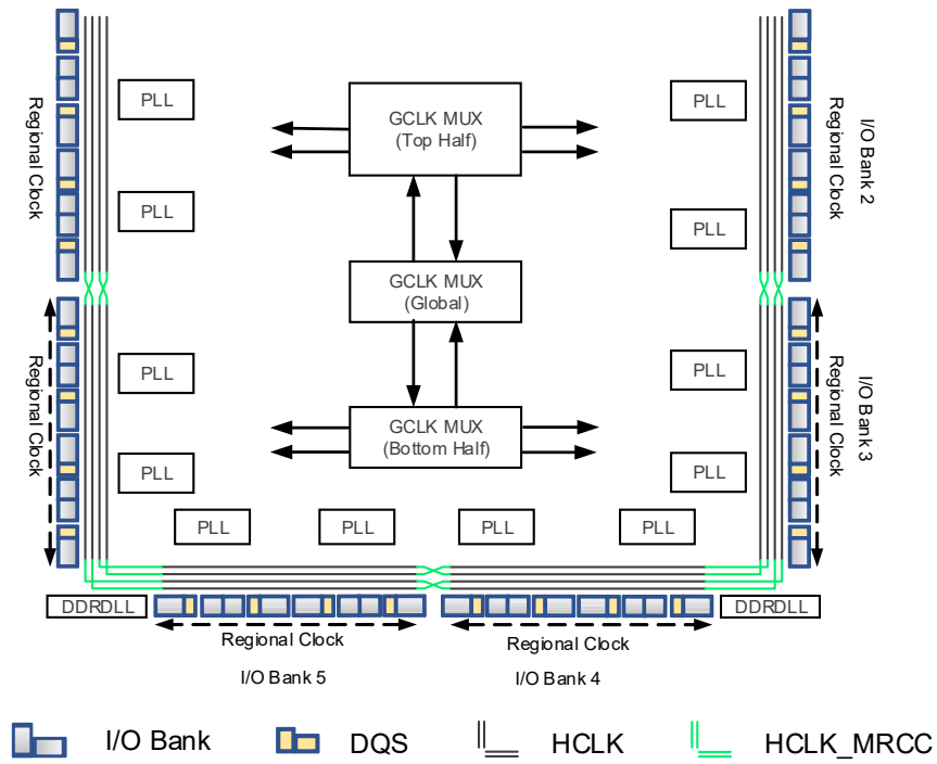
图 2-17 器件时钟资源(GW5AT-75)
