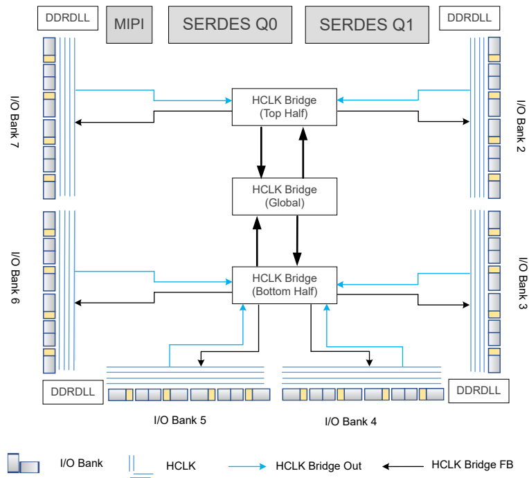
图 2-21 HCLK 示意图(GW5AT-75)
