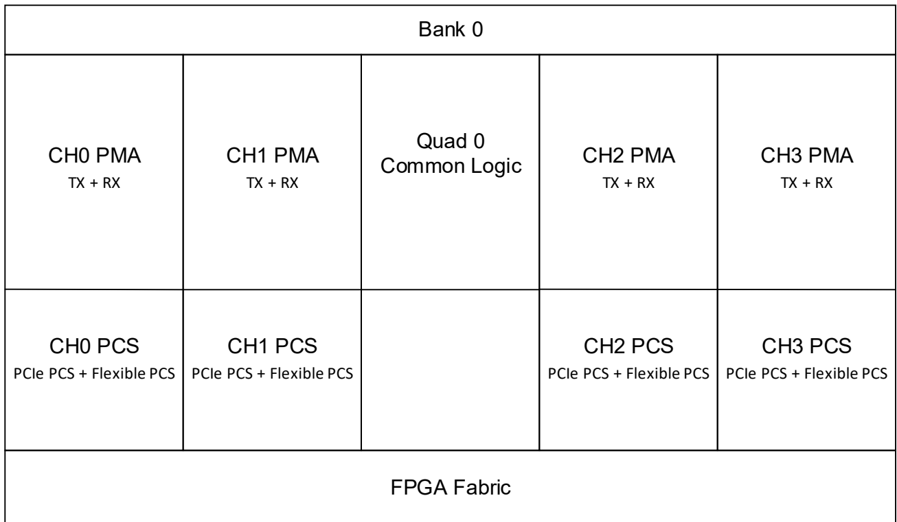
图 2-15 Gigabit Transceiver 结构示意图
