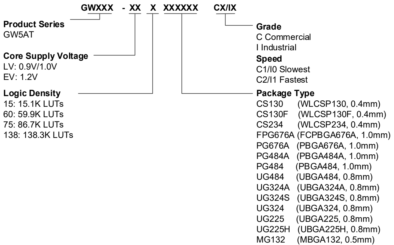
图 4-2 器件命名方法示例-Production
