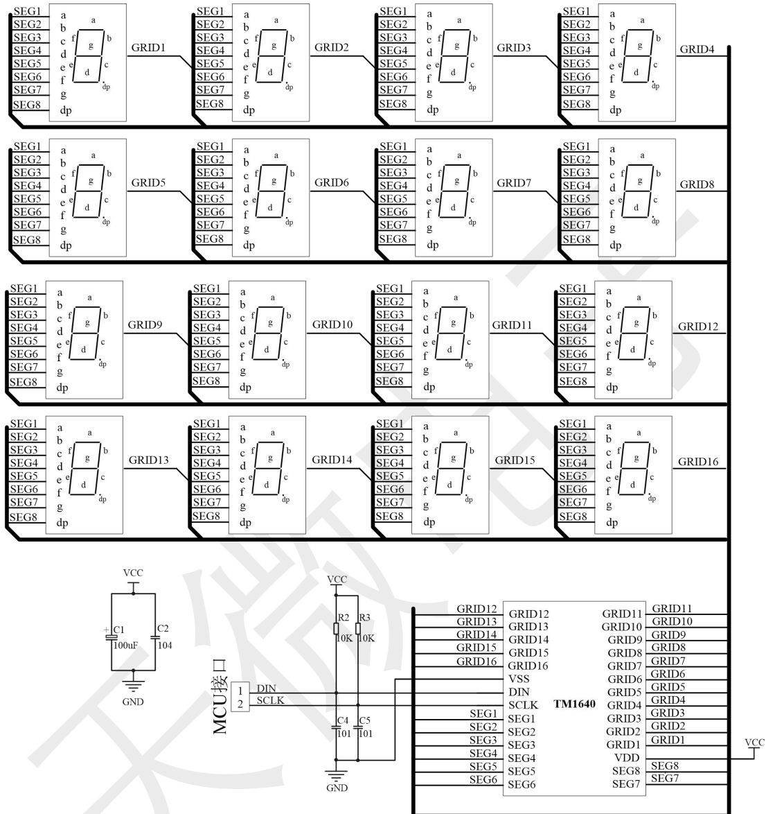
TM1640 驱动共阴极数码管硬件电路图:
