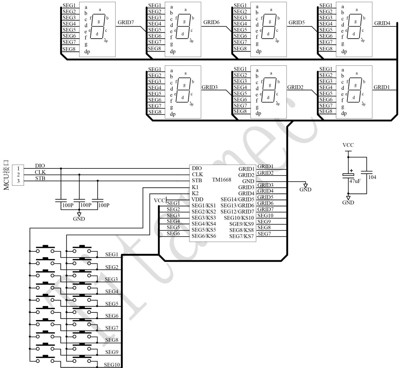
TM1668驱动共阴数码屏硬件电路图（18）
