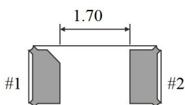
Bottom View(1)
