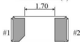
Bottom View(2)
